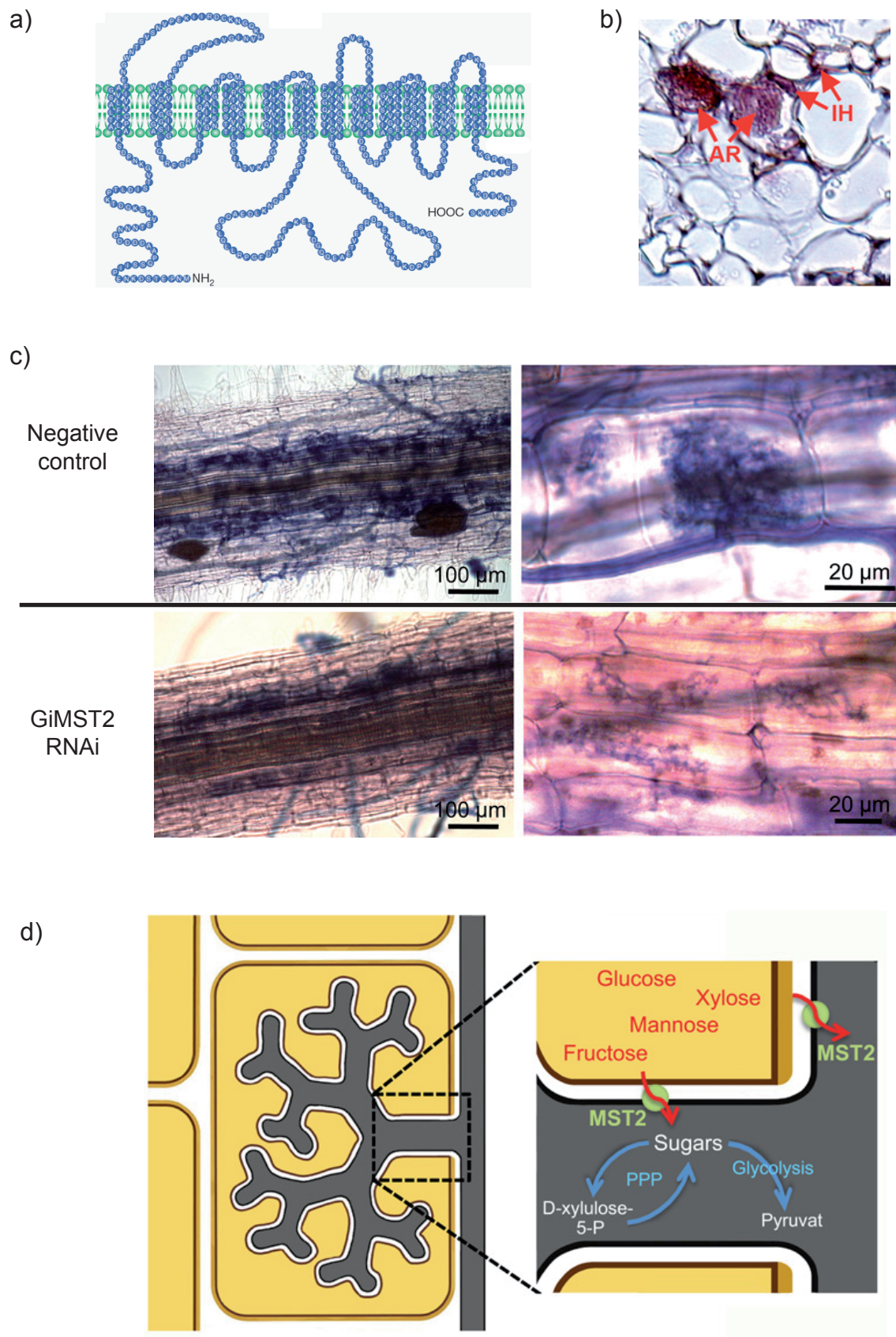
Fig 26. Glomeromycotan sugar transporters (Schüßler et al. 2006; Helber et al. 2011)
