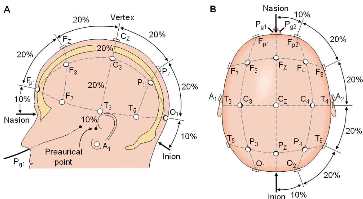
Figure 12 : Placement des électrodes EEG selon le Système International 10-20 ( Malmivuo & Plonsey, 1995 ).
